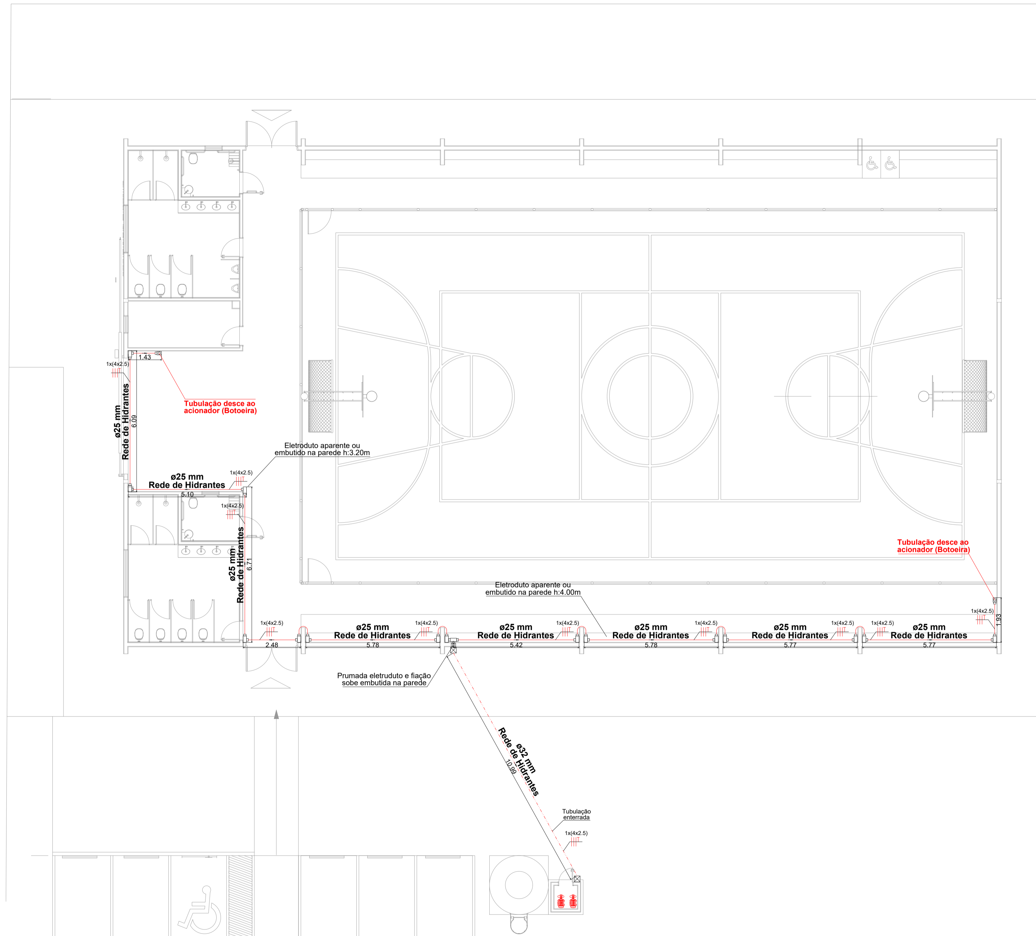
1 Planta baixa - Infraestrutura rede de hidrantes ESCALA: 1:100
