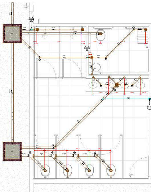
1 PLANTA BAIXA - ESGOTO SANITÁRIO - WC FEM. 1:25
