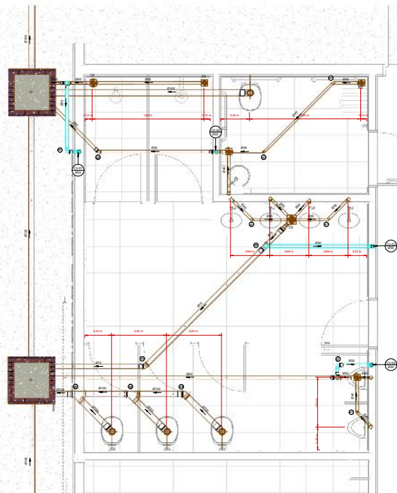
2 PLANTA BAIXA - ESGOTO SANITÁRIO - WC MASC. 1:25
