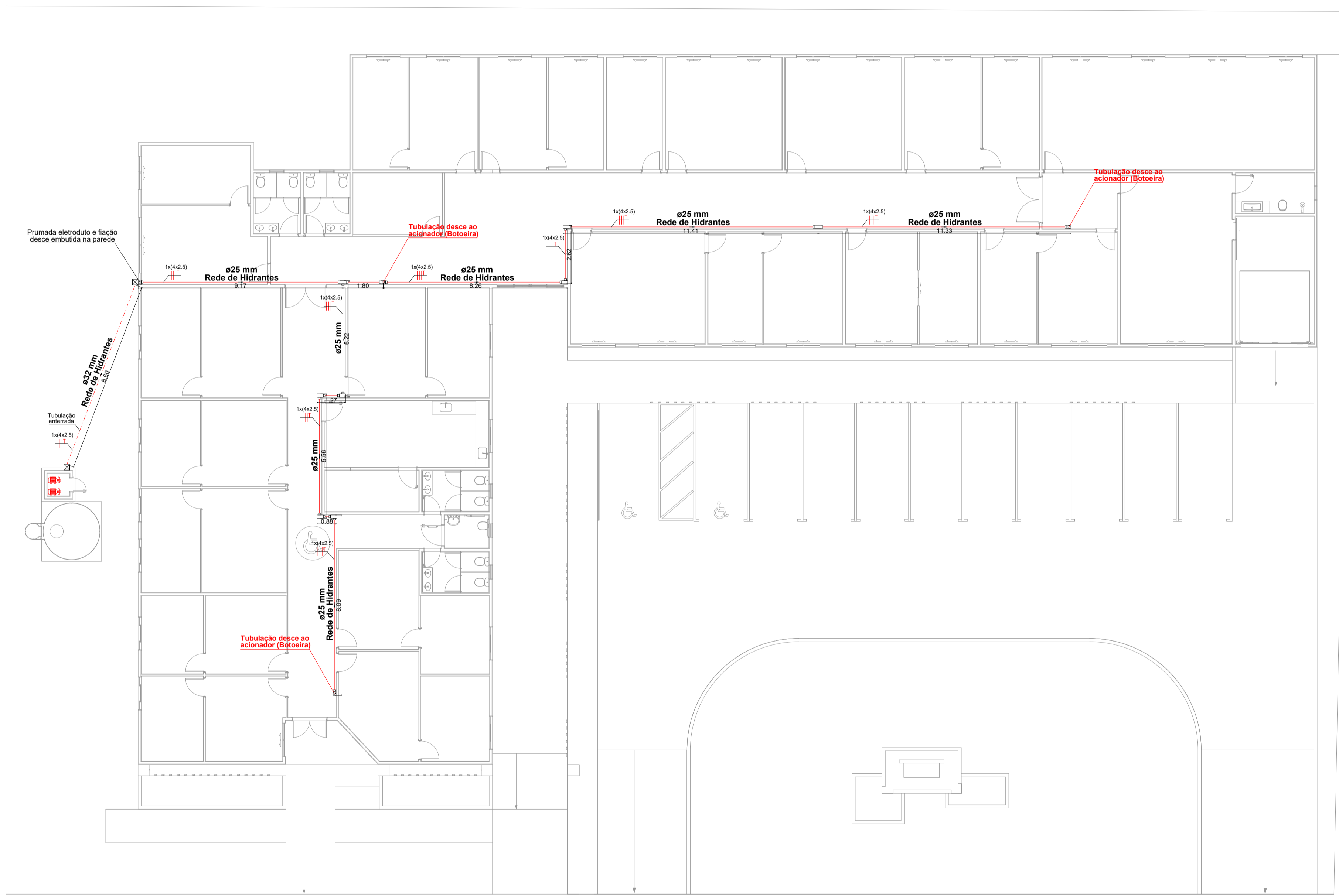
1 Planta baixa - Infraestrutura rede de hidrantes ESCALA: 1:125
