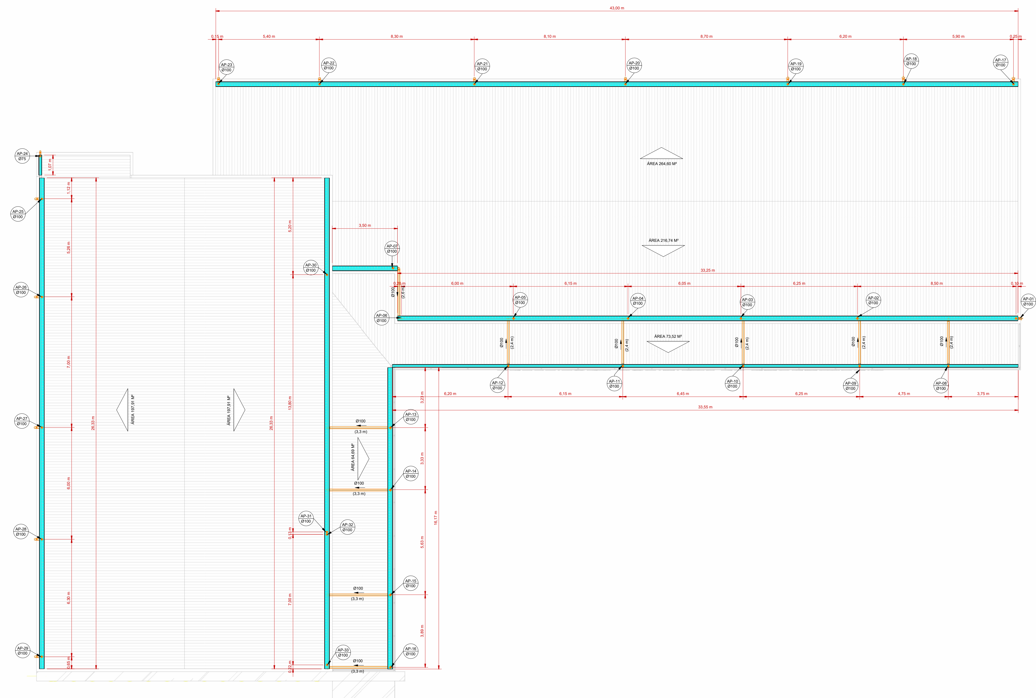
1 DRENAGEM PLUVIAL - COBERTURA 1 : 100
