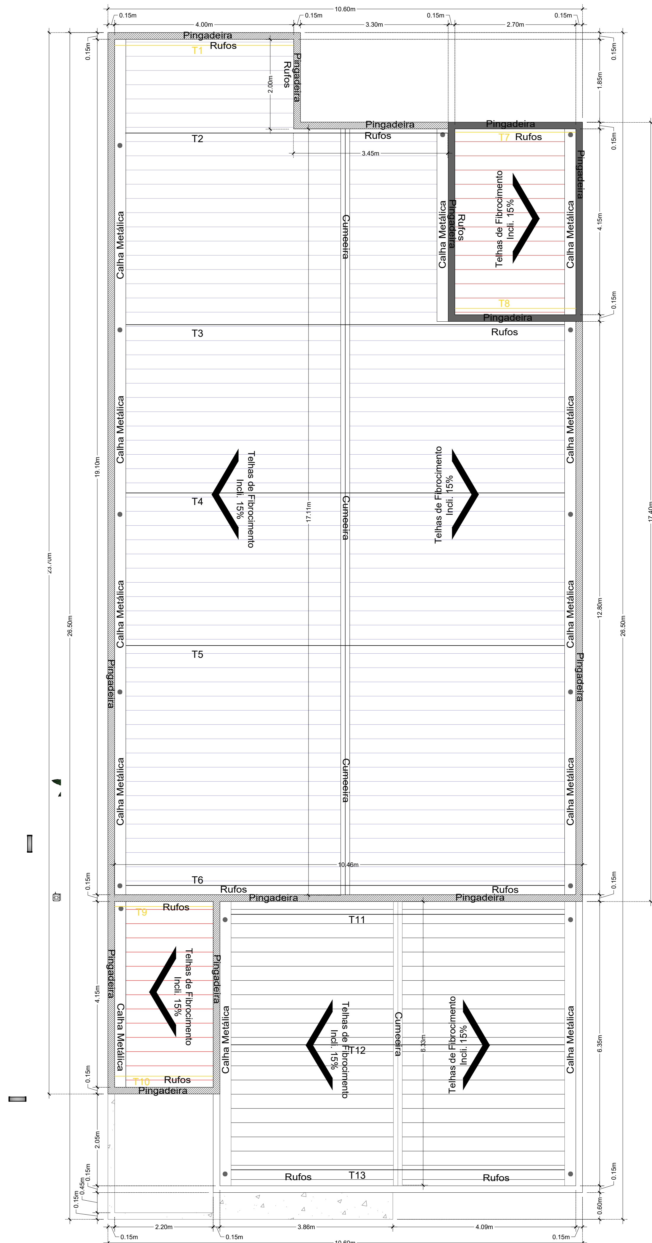
2 PLANTA DE COBERTURA E = 1 : 50
