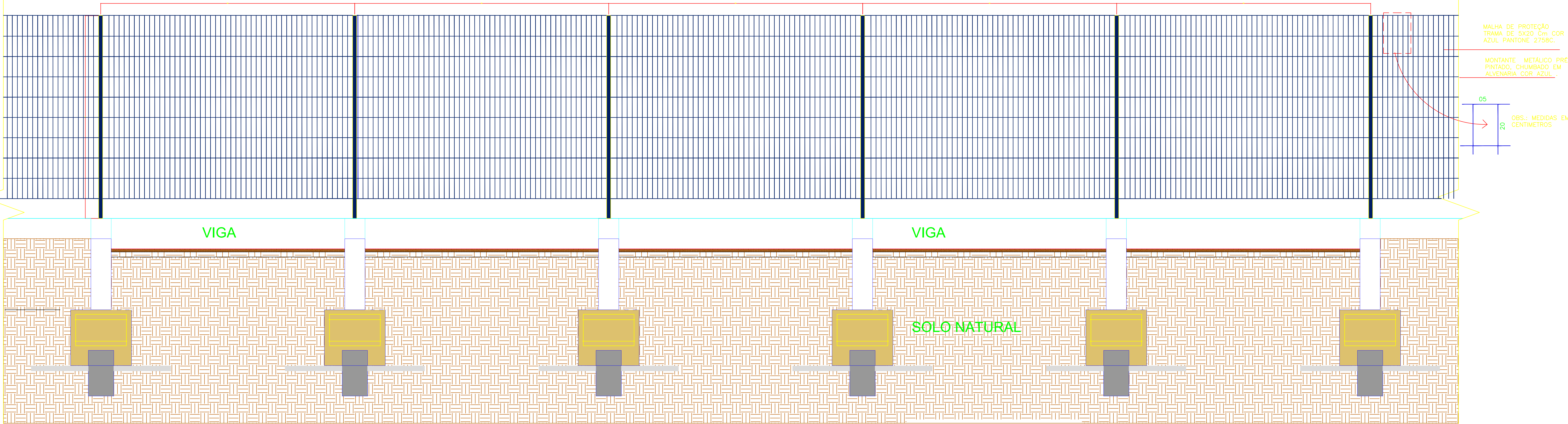
2. CORTE LONGITUDINAL Esc: 1/50
