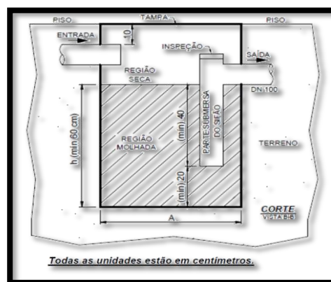
Figura 4. Detalhe da Caixa de Gordura
