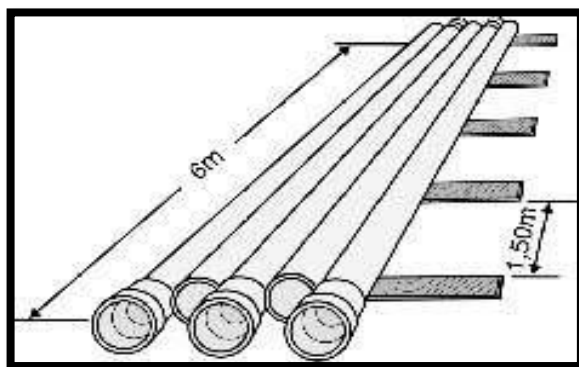
Figura 13. Camada cruzada
