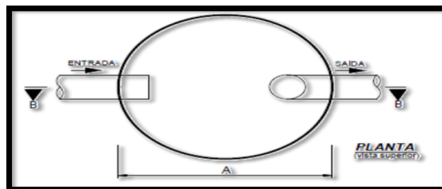
Figura 3. Detalhe da Caixa de Gordura
