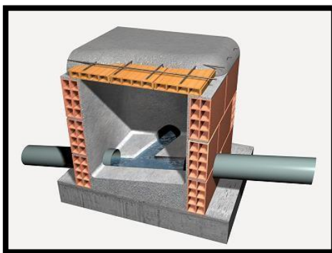
Figura 2. Execução do fundo das caixas de passagem
