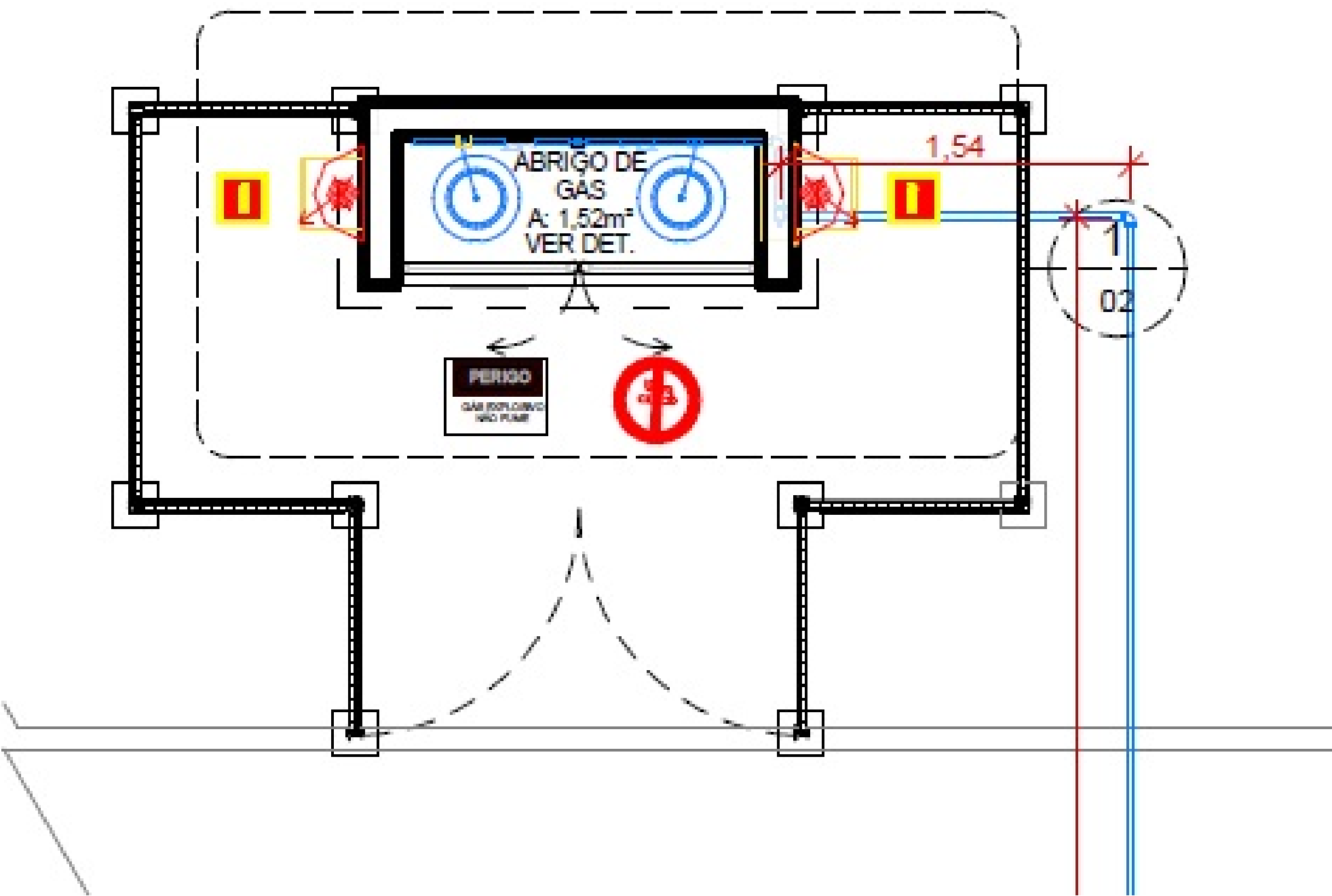
DETALHE DA CASA DE GÁS
